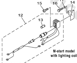
RECTIFIER KIT
